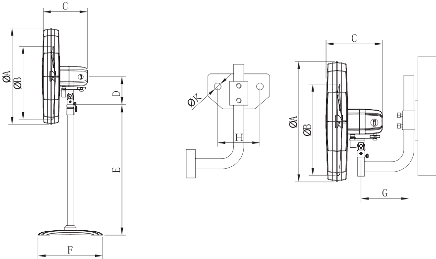
外形尺寸图 Outline dimensions
