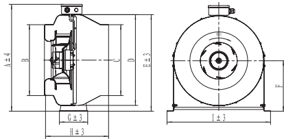
CDF20-66E、CDF25-66E、CDF31-66E CDF20-66A、CDF25-66A、CDF31-66A
