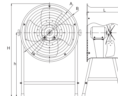
外形尺寸图 Outline dimensions
