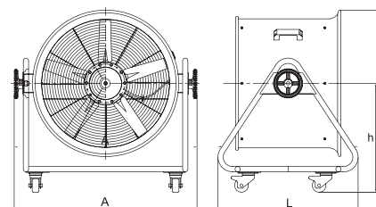
外形尺寸图 Outline dimensions
