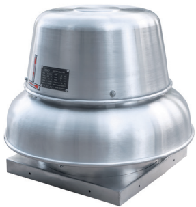
Direct Drive Models:RC-A: 200、260、320、360、400、450、500 Air volume:728-9901m³/h Total pressure:44-335Pa
