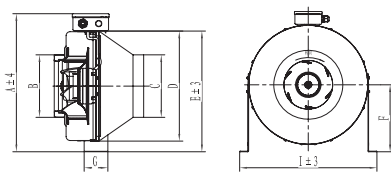
CDF15-45E、CDF16-45E CDF15-45A、CDF16-45A
